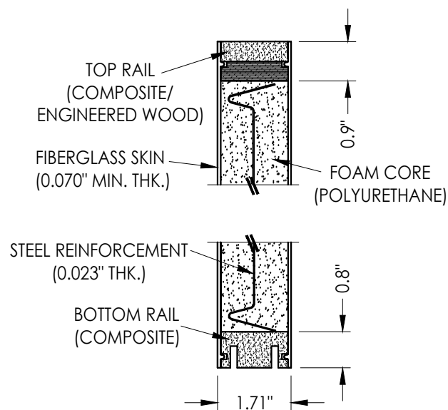
SECTION D-D
