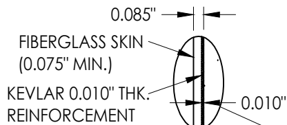
DOOR SKIN DETAIL
